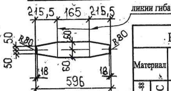
Развертка поз.1
